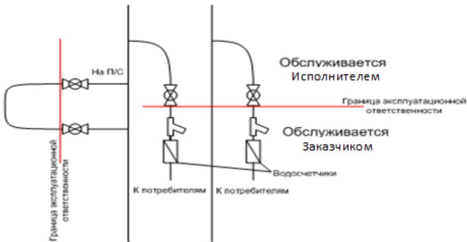
Трубопровод ГВС Трубопровод ХВС
